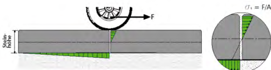
Abbildung 9: Unterschiedliche Lastabtragung im Bereich der Stoßfuge bei einer Platte mit ausreichender Steinhöhe [3]
