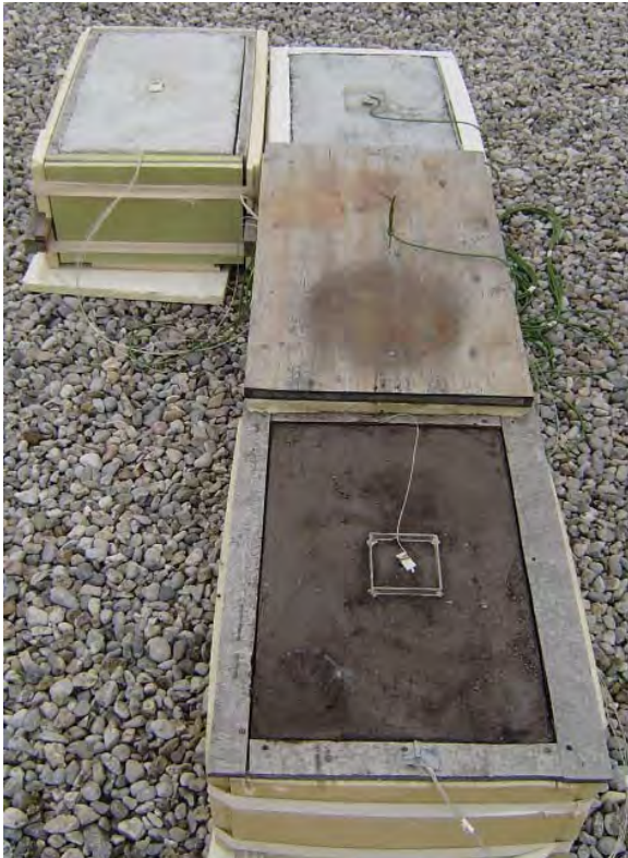
Abbildung 4: Versuchskörper zur Messung des Erwärmungsverhaltens am Dach des Institutsgebäudes der Vereinigung der österreichischen Zementindustrie [Foto VÖZFI]
