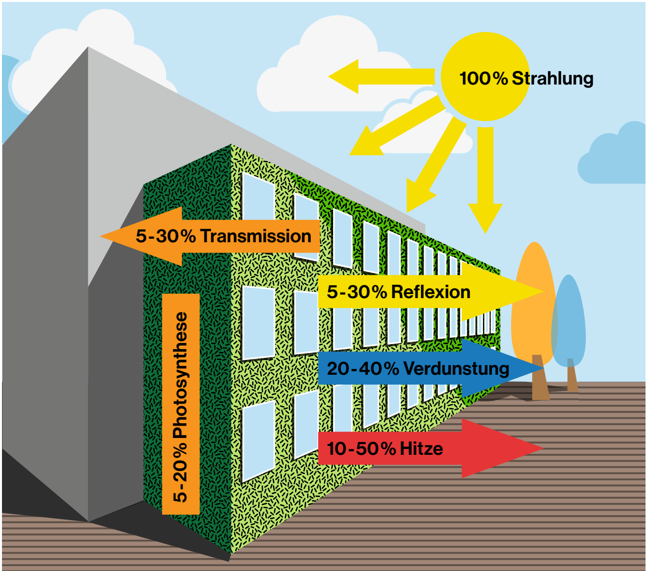
Energiebilanz einer begrünten Fassade (KRUSCHE et.al., 1982)
